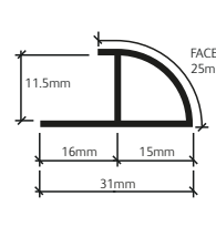
Quadrant Trim
