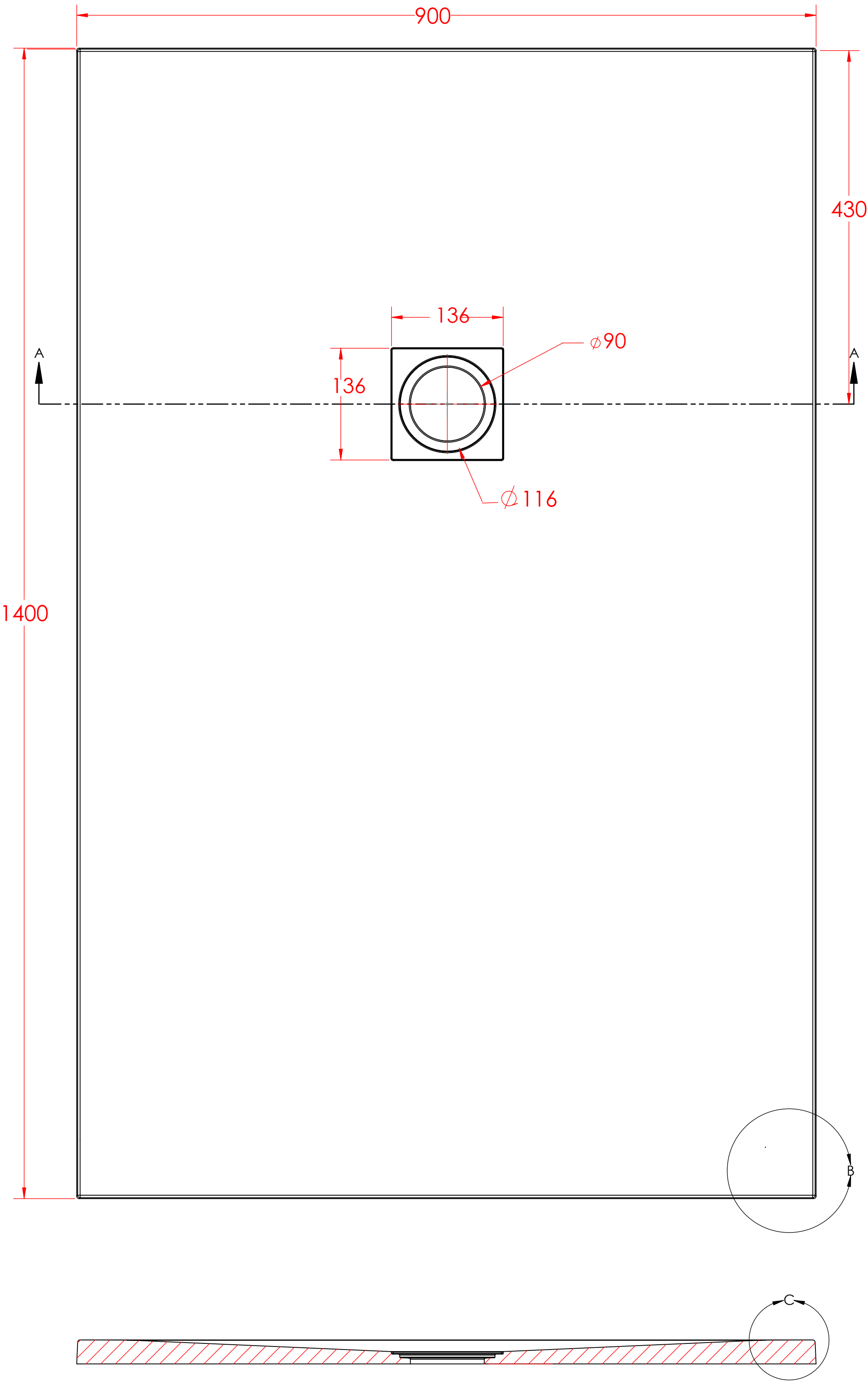
SECTION A-A SCALE 1 : 4
