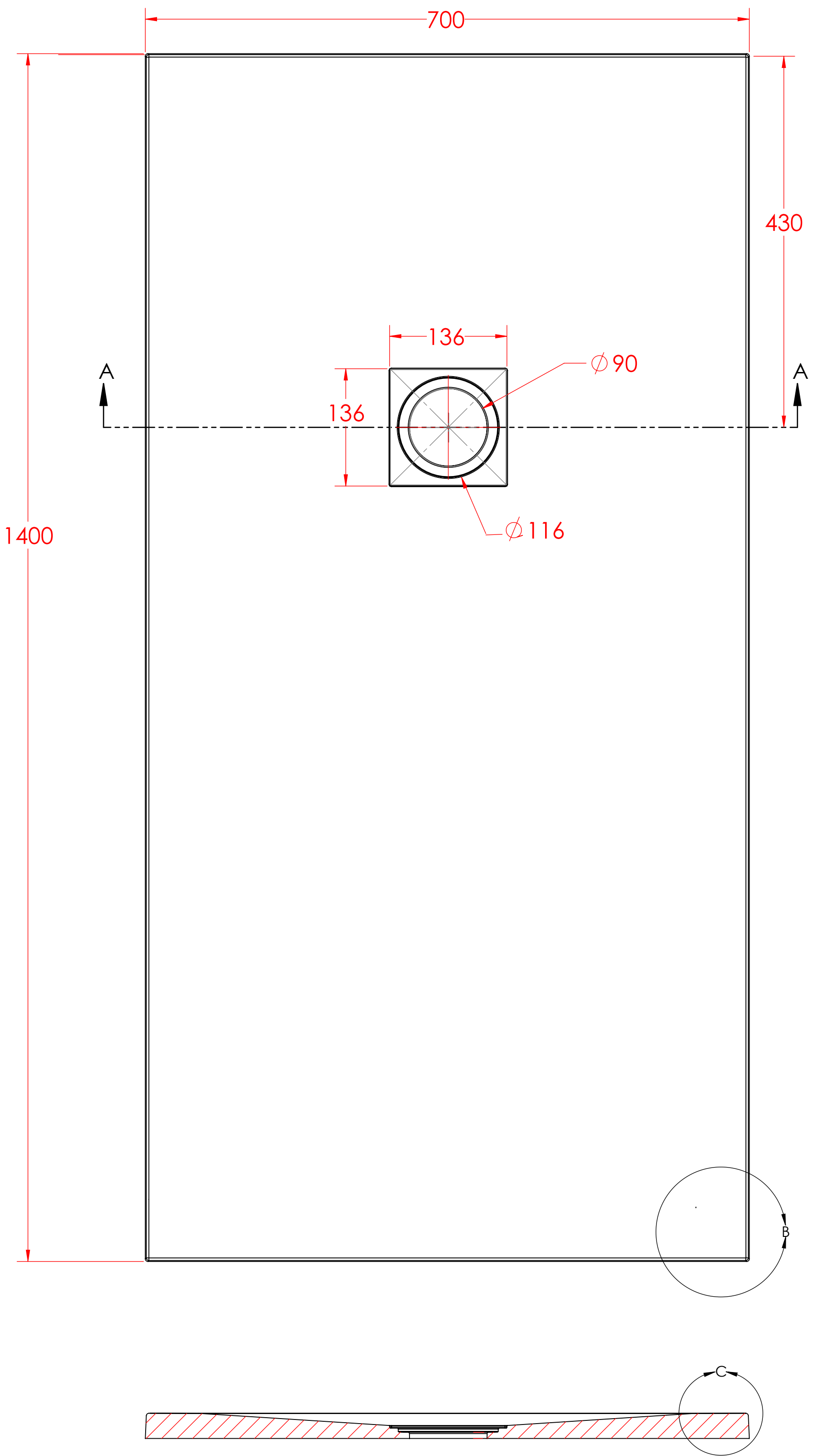
SECTION A-A SCALE 1 : 4
