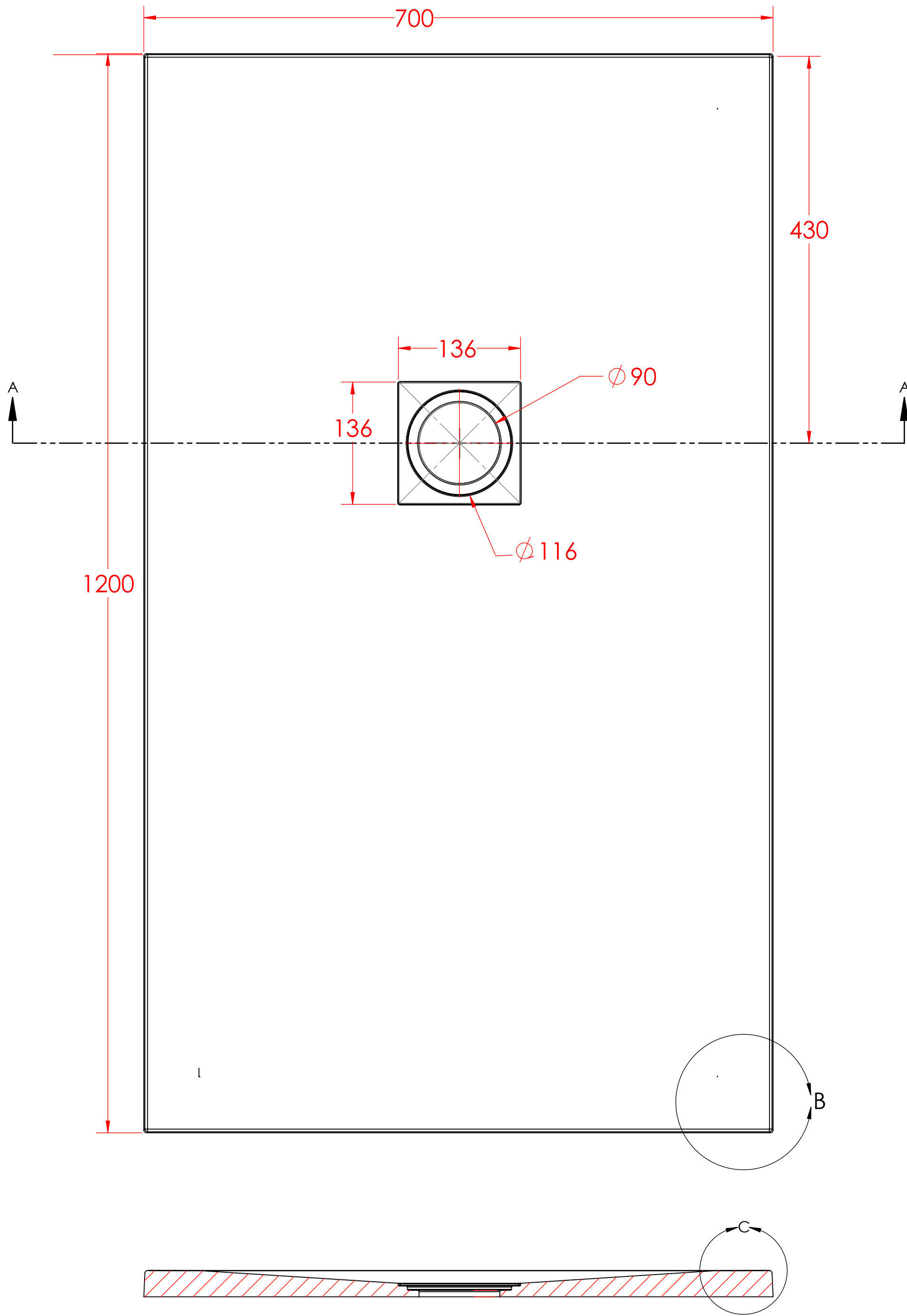
SECTION A-A SCALE 1 : 4
