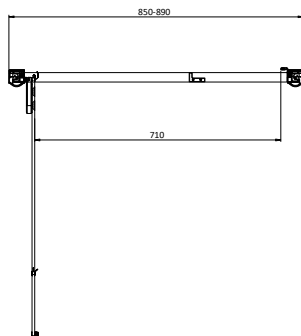
Hinge door 900
