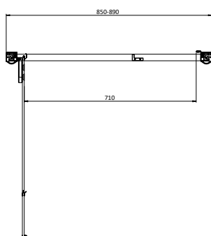
Hinge door 900
