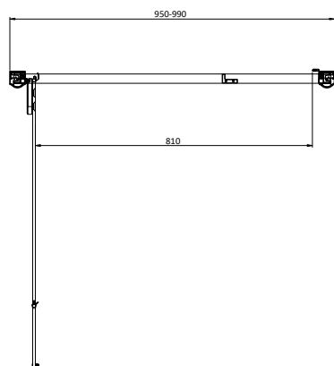
Hinge door 1000
