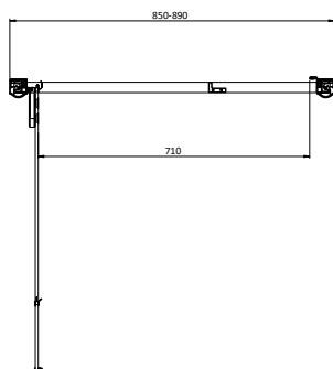
Hinge door 900
